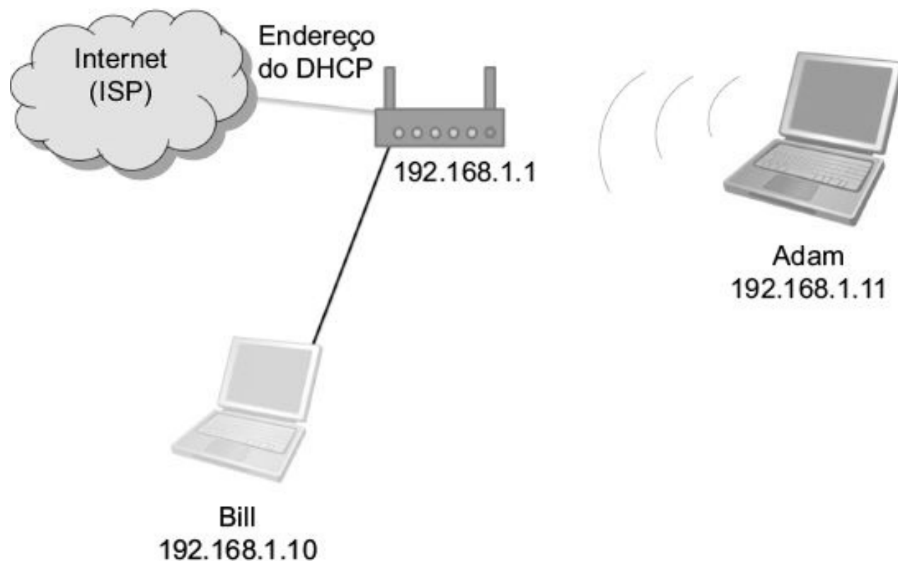
Figura 4.3 – Exemplo de um pequeno segmento de rede.
